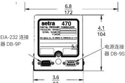
正面视图
