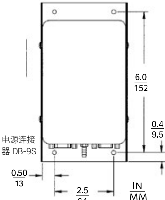
顶部视图
