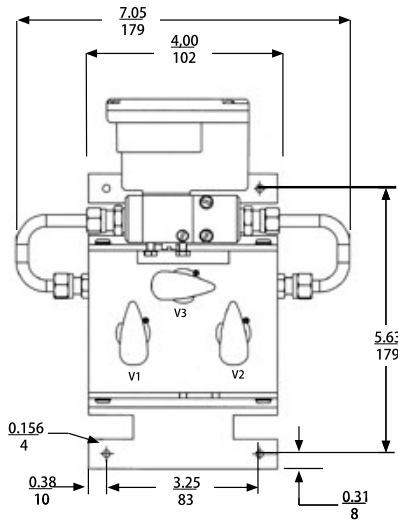
主视图
