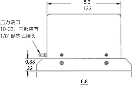
侧面视图
